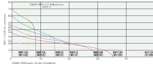
■ スタンダードロータリー 回転数/トルク曲線 (モーター単体のデータ) Speed/Torque Curve (data for a motor component)
